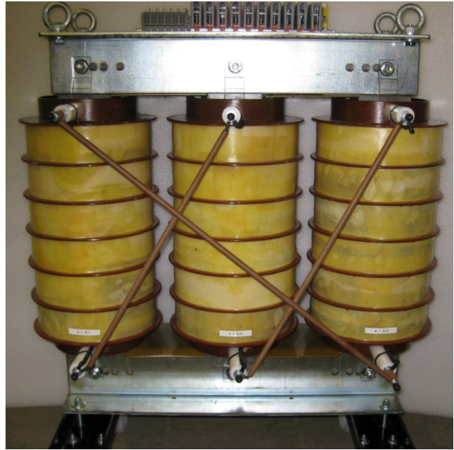
Blas magnetisation transformer 50 KVA
